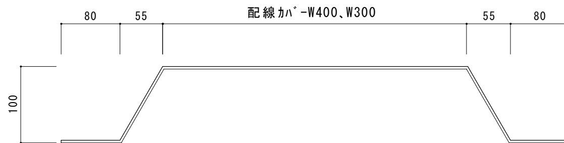
配線カハ参考図 S=1/5
